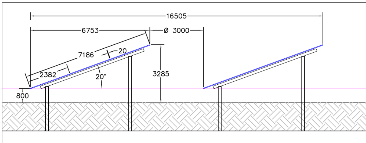
Abbildung 8: Systemschnitt Modultische mit Seitenansicht (alle Maße in Millimeter), Quelle: solargrün GmbH, 2024
