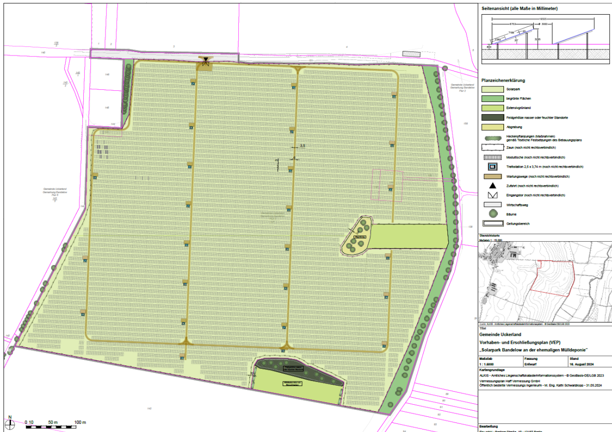
Abbildung 7: Vorhaben- und Erschließungsplan, Quelle: FIRU mbH 2024, Datengrundlage E4R - Engineers for Renewables GmbH (2024): Modulbelegungsplan - Entwurfsplanung
